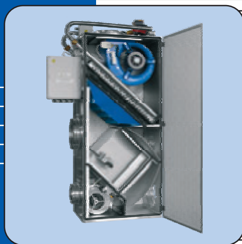
Vytápěcí a větrací bazénová jednotka s rekuperací tepla DUPLEX RDH
